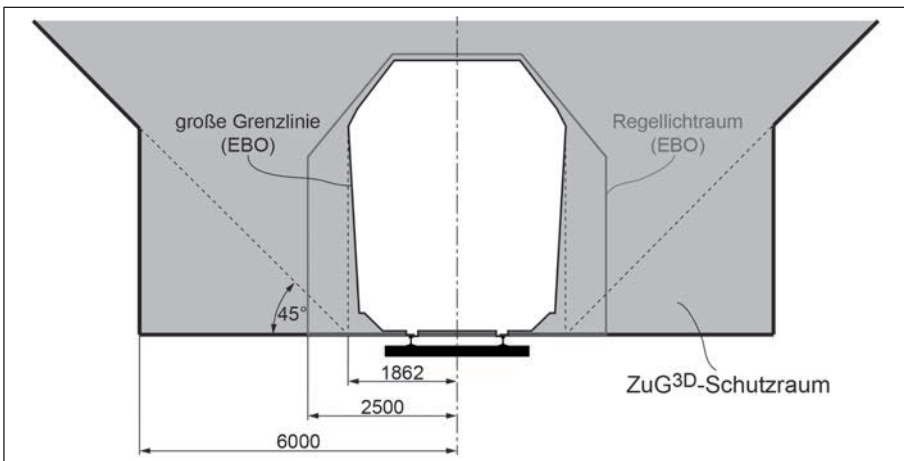
Abb. 4: Beispiel des ZuG 3D -Schutzraums als Kombination von U- und V-Profil
